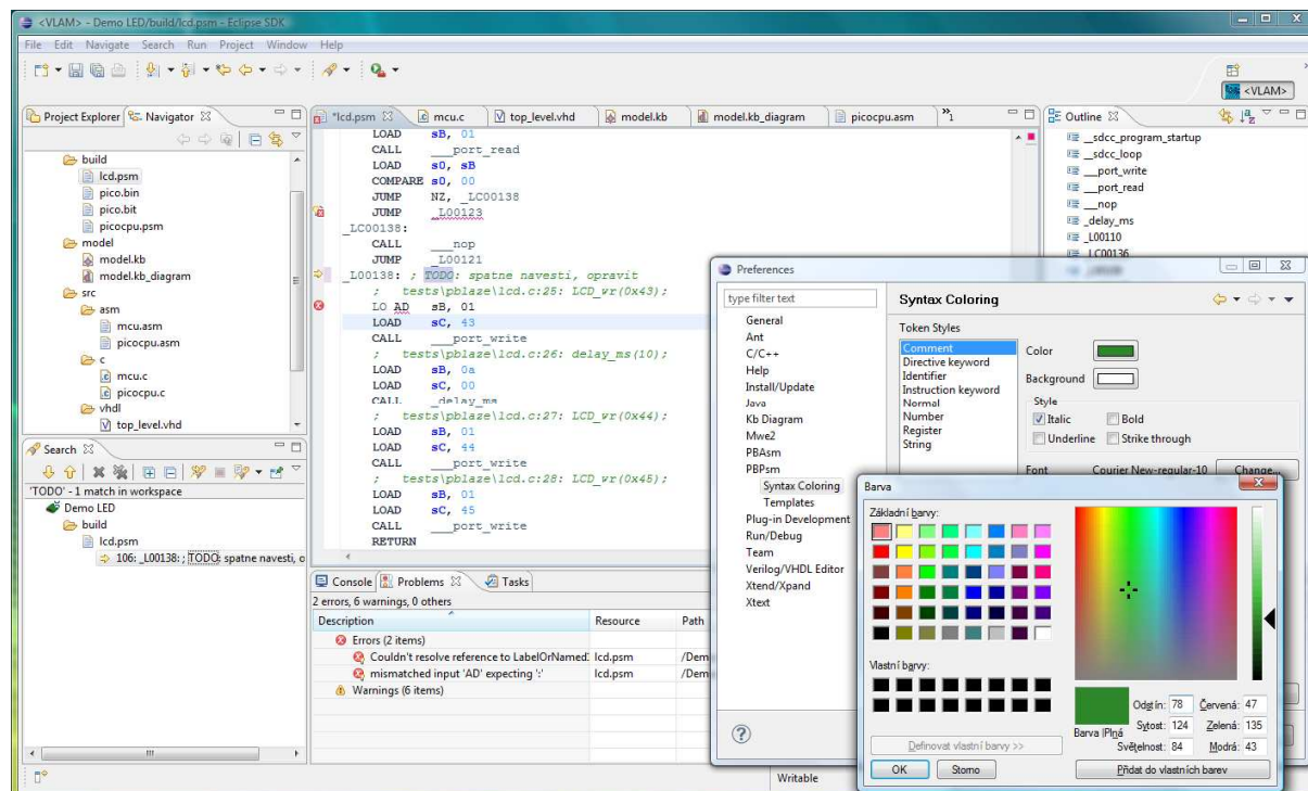
Obrázek 21: Ukázka editoru PBPsm včetně ukázky konfigurace zvýrazňování syntaxe (dialog Preferences a Barva )
