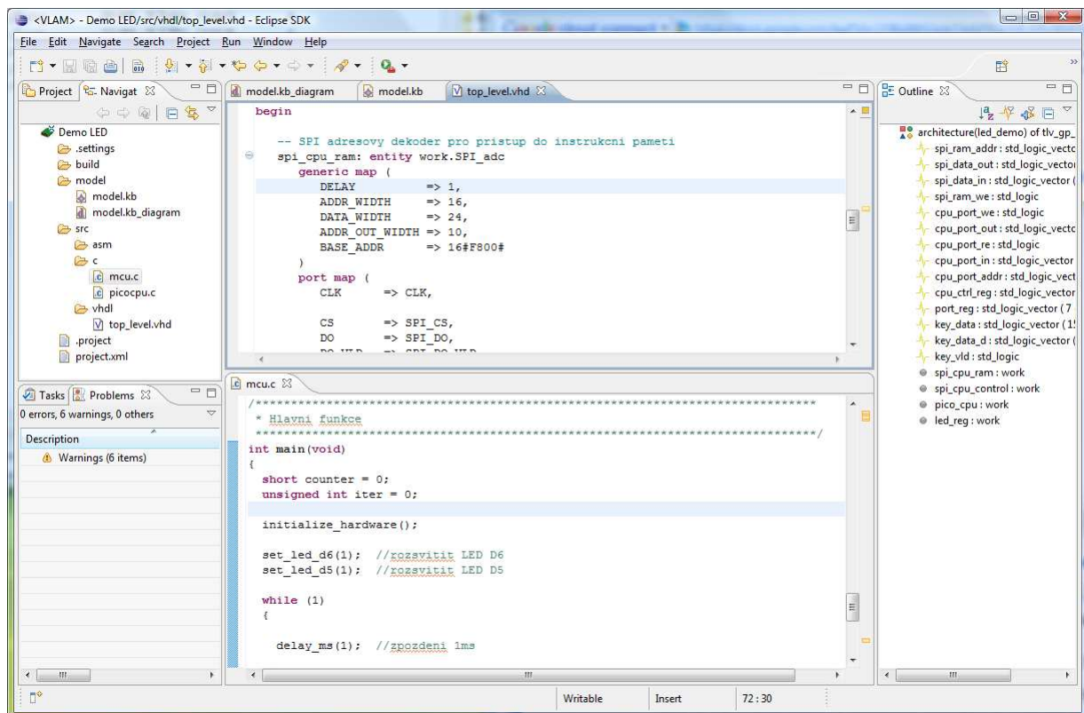
Obrázek 29: Vygenerované HDL (horní prostřední panel) a kód pro mikrokontrolér (dolní prostřední panel)
