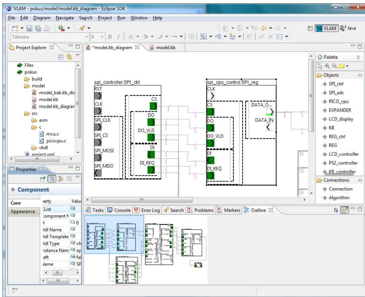
Obrázek 15: Ukázka mnoha pohledu otevřených v perspektivě VLAM
