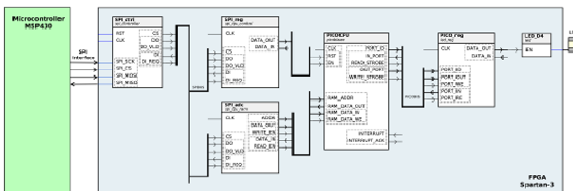
Obrázek 25: Schéma návrhu hardware pro FPGA
