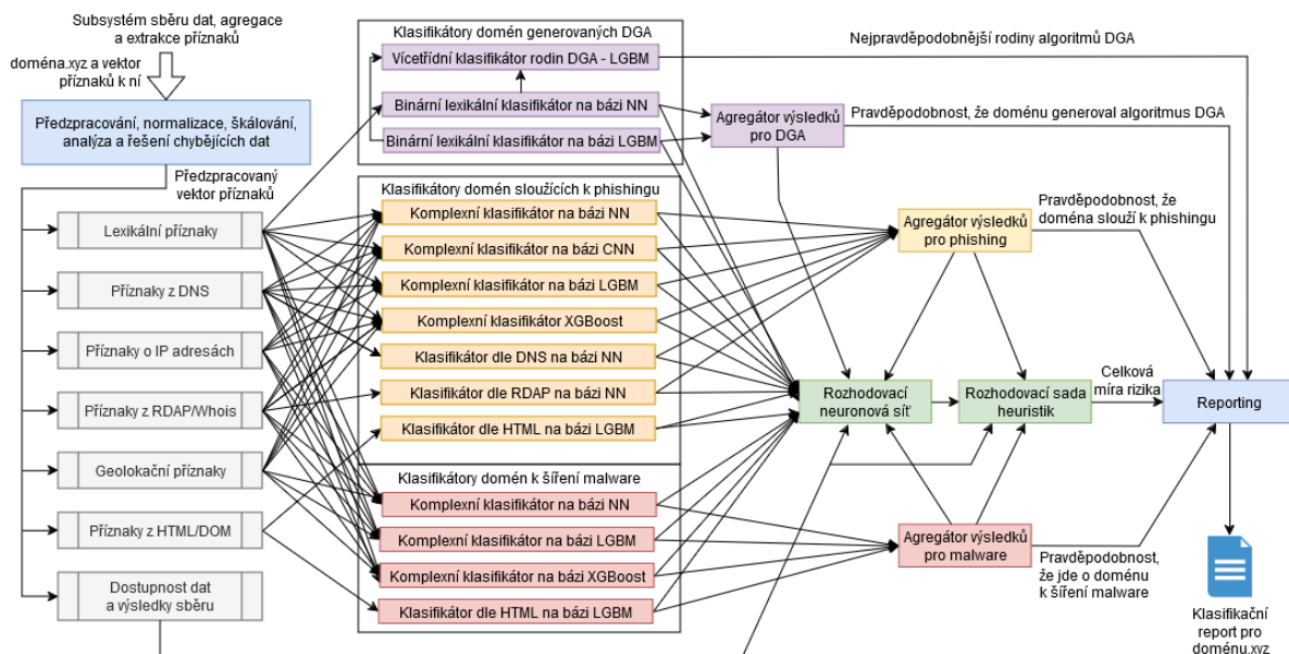
Obrázek 11: Architektura klasifikační pipeline
